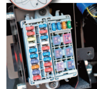
Quadro fusibili con legenda
